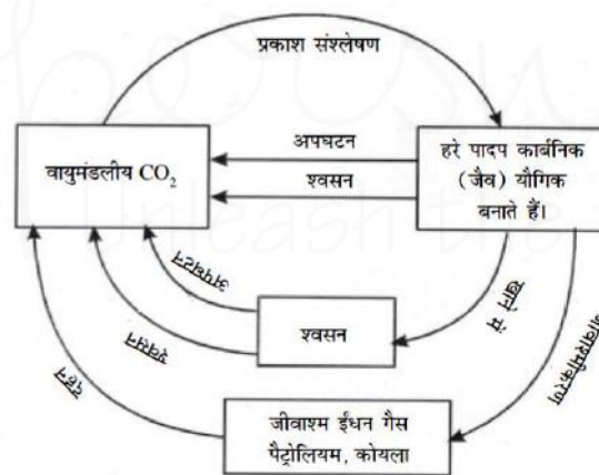
चित्र 5.6: कार्बन चक्र
