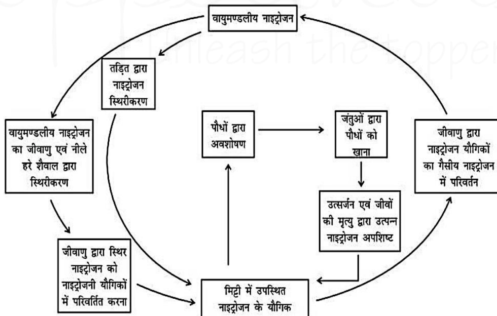
चित्र 2.10 : नाइट्रोजन चक्र।
