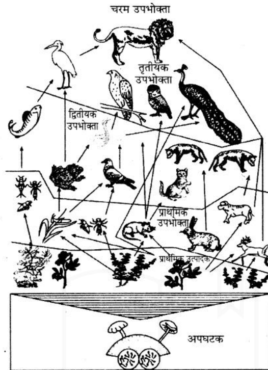
चित्र 40.4 : एक स्थलीय पारिस्थितिक तंत्र में खाद्य जाल।
