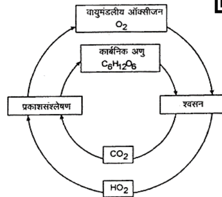
चित्र—प्रकृति में ऑक्सीजन चक्र
