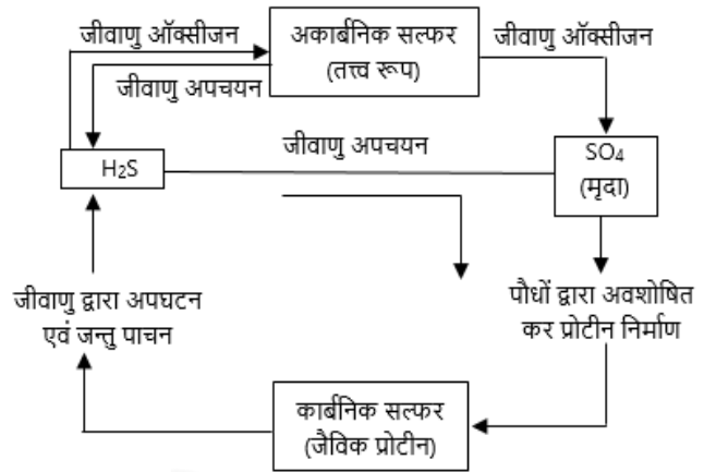
चित्र - प्रकृति में सल्फर चक्र
